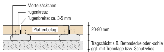
Plattenverlegung auf Mörtelsäckchen (Fugen offen)
